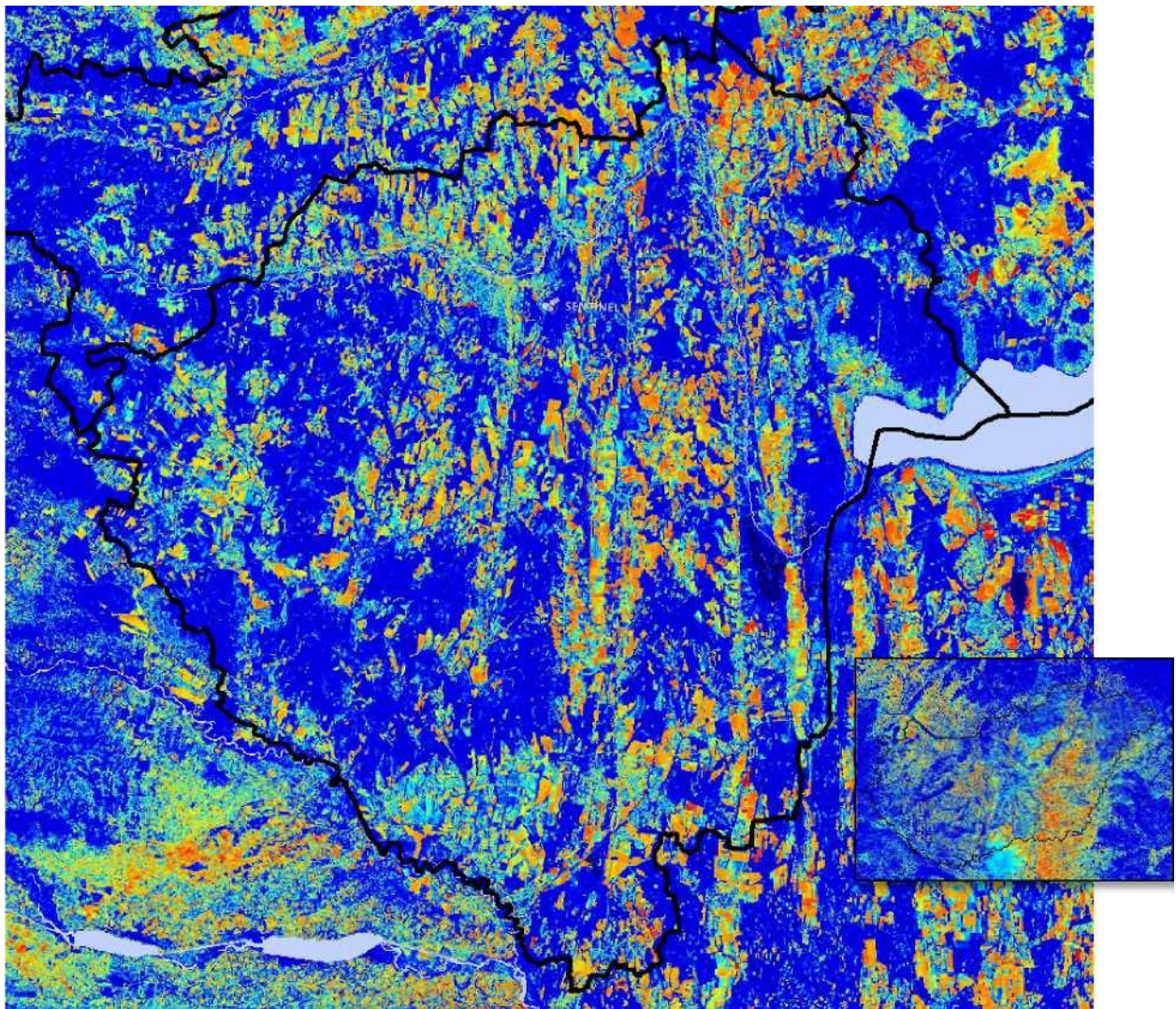
7. ábra Talajok nedvesség index (Sentinel 2 műhold - 2017.08.31.)
